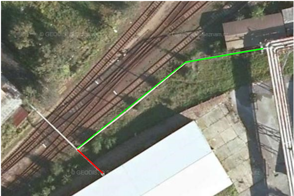
Foto 1 : letecký pohled na mosty A1 U 18 P (zeleně) a A1 S18 P (červeně), bíle A1 S19 P
