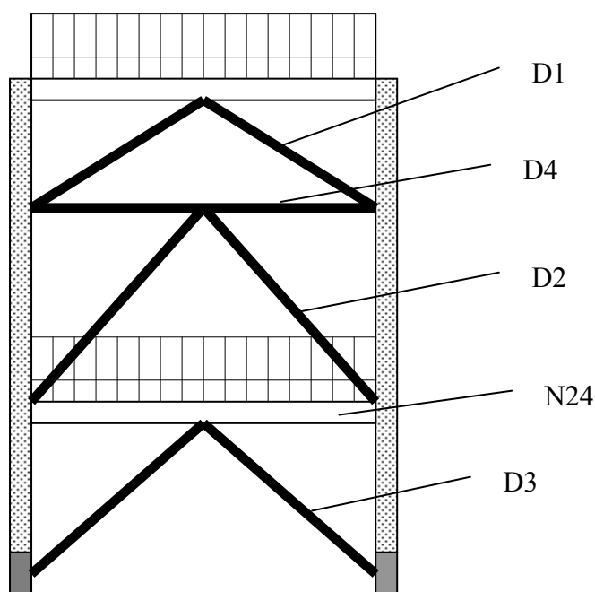
Konstrukční schéma výměny dílů sloupová 4 – zadní pohled (od budovy)
