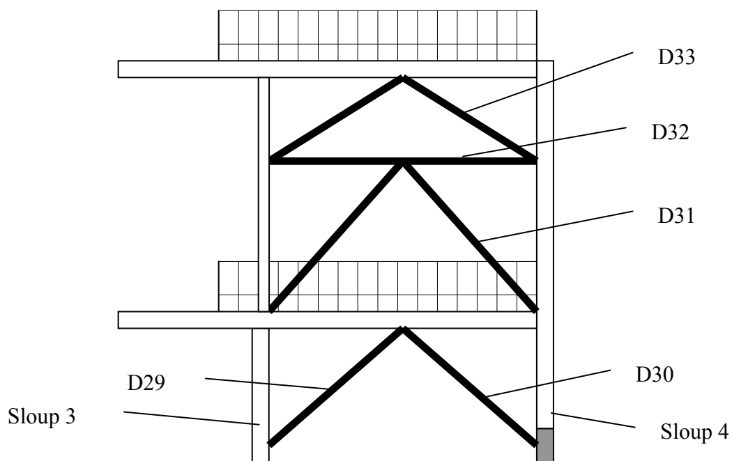
Konstrukční schéma výměny dílů mezi sl. 3 a 4 (boční pohled)
