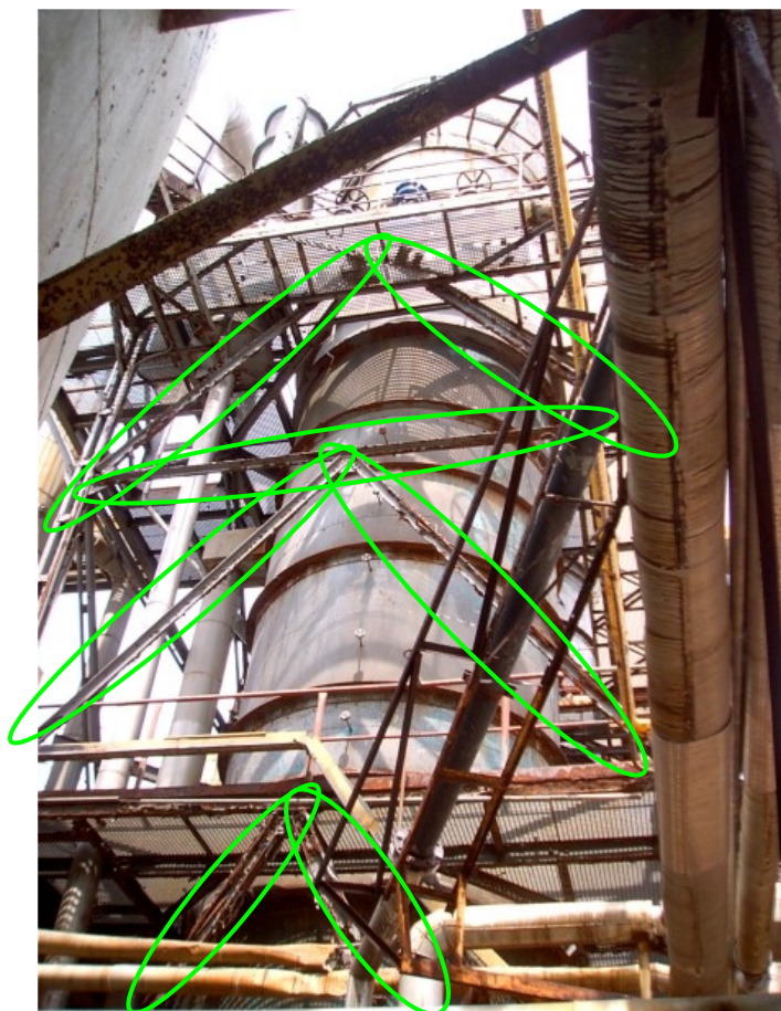
Foto 3 : Pohled na konstrukci linky č. 2 z boku od linky č.1 – díly k výměně označeny
