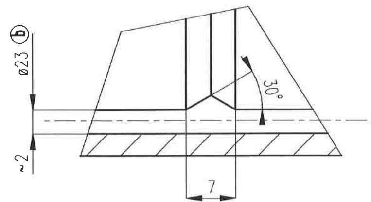
DETAIL A ⓐ M 2:1
