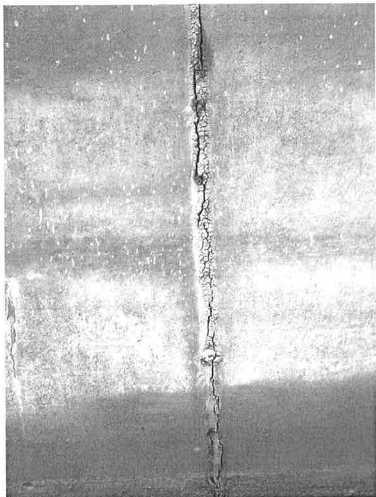
foto č. 3 – D1760: vypráskaná dilatační spára
